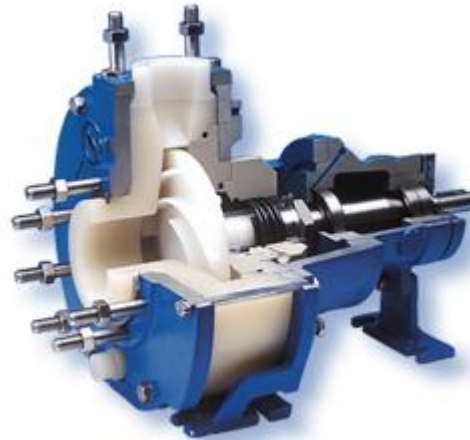
BOMBA CENTRIFUGA HORIZONTAL EN PP
